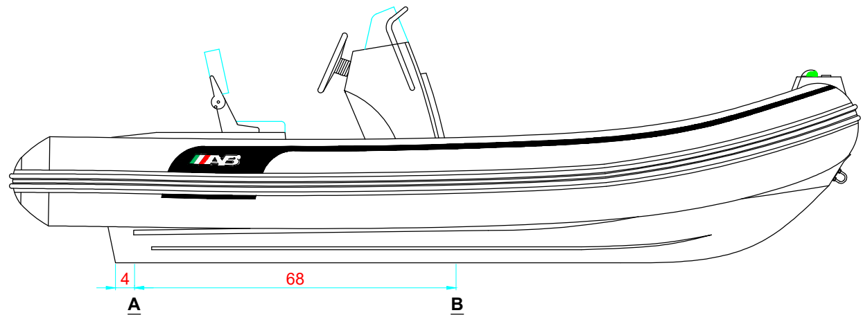
LONGITUDINAL PROFILE VISTA LATERAL
