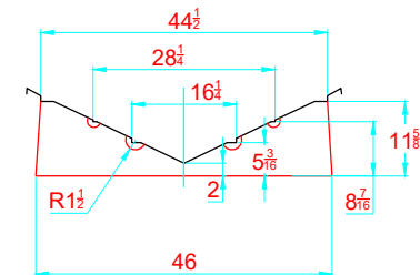
TRANSVERSAL SECTION "B" SECCION TRANSVERSAL "B"
