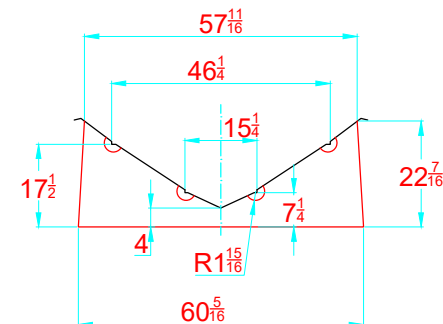
TRANSVERSAL SECTION "B" SECCION TRANSVERSAL "B"
