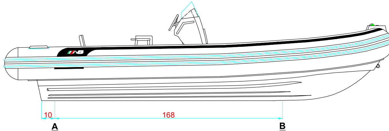
LONGITUDINAL PROFILE PERFIL LONGITUDINAL
