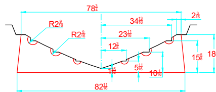
TRANSVERSAL SECTION "B" SECCION TRANSVERSAL "B"
