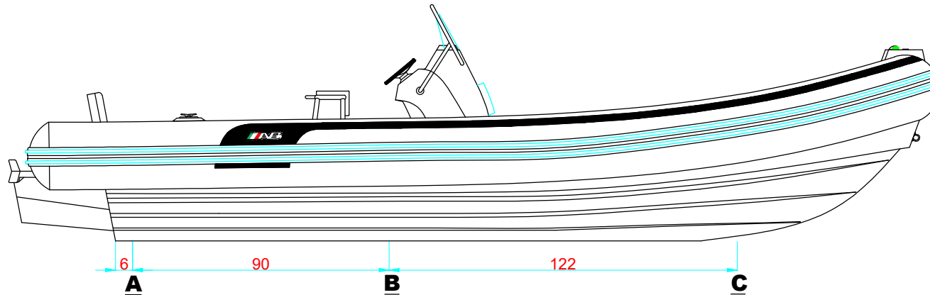
LONGITUDINAL PROFILE VISTA LATERAL
