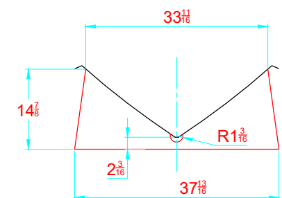
TRANSVERSAL SECTION "B" SECCION TRANSVERSAL "B"
