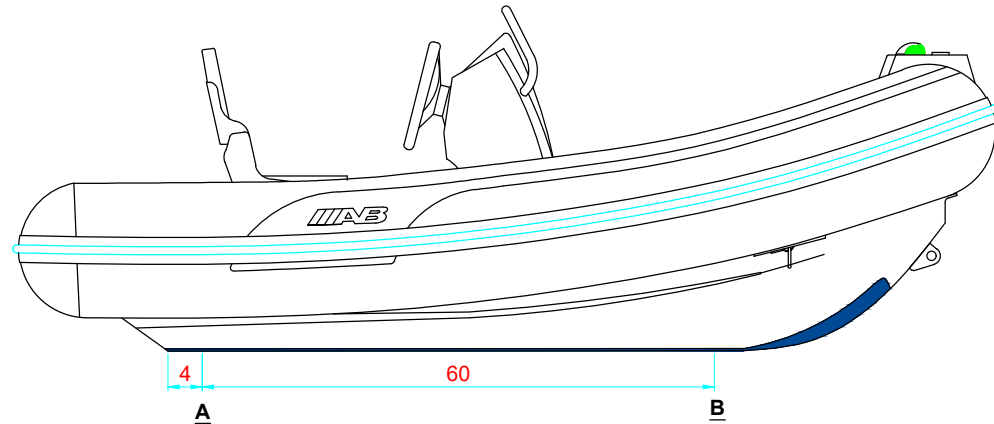
LONGITUDINAL PROFILE PERFIL LONGITUDINAL
