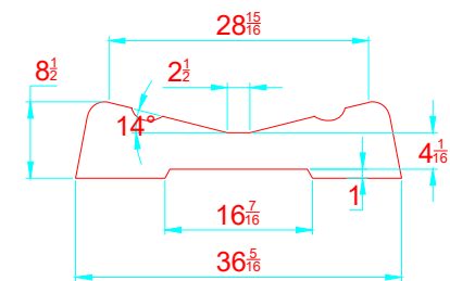
TRANSVERSAL SECTION "B" SECCION TRANSVERSAL "B"
