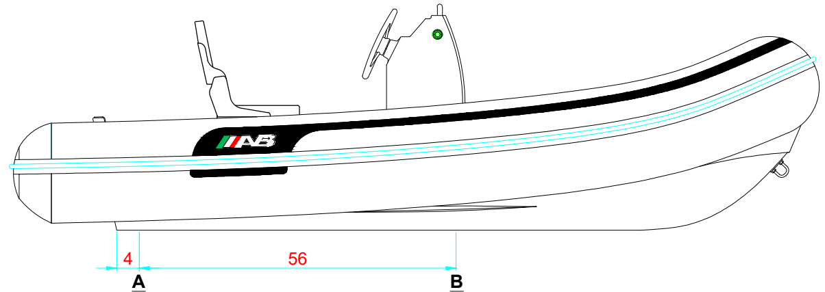
LONGITUDINAL PROFILE VISTA LATERAL
