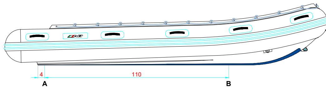
LONGITUDINAL PROFILE PERFIL LONGITUDINAL
