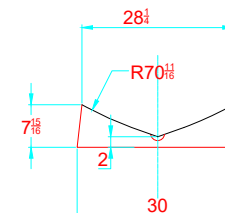
TRANSVERSAL SECTION "B" SECCION TRANSVERSAL "B"
