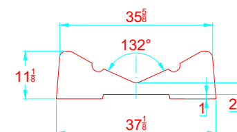
TRANSVERSAL SECTION "B" SECCION TRANSVERSAL "B"
