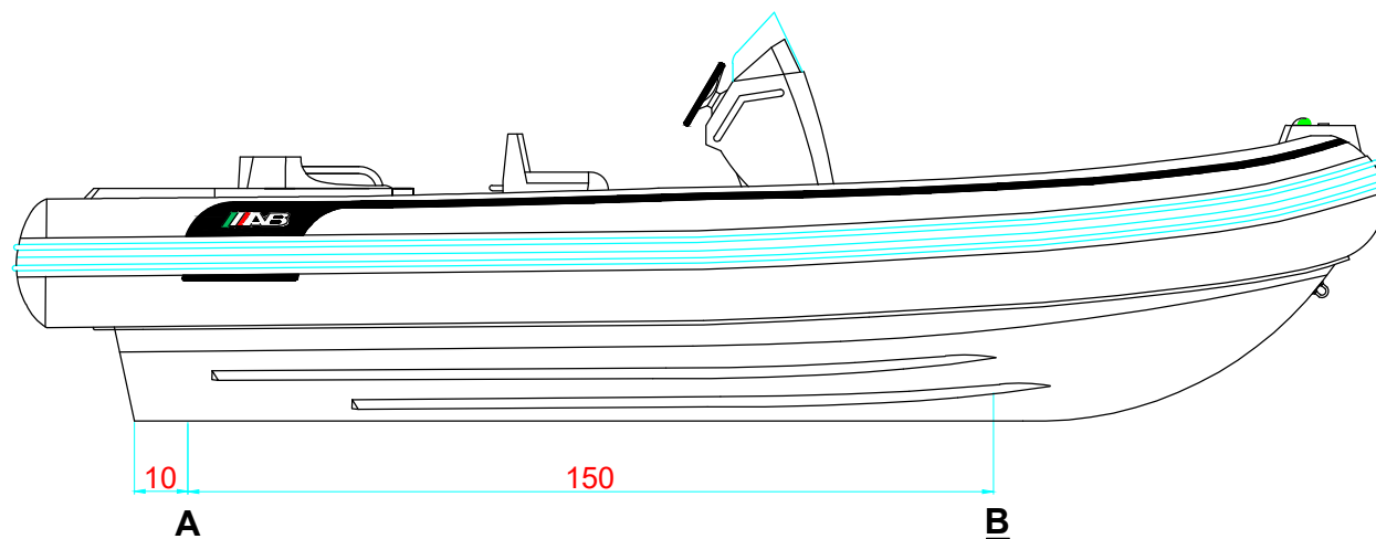
LONGITUDINAL PROFILE PERFIL LONGITUDINAL
