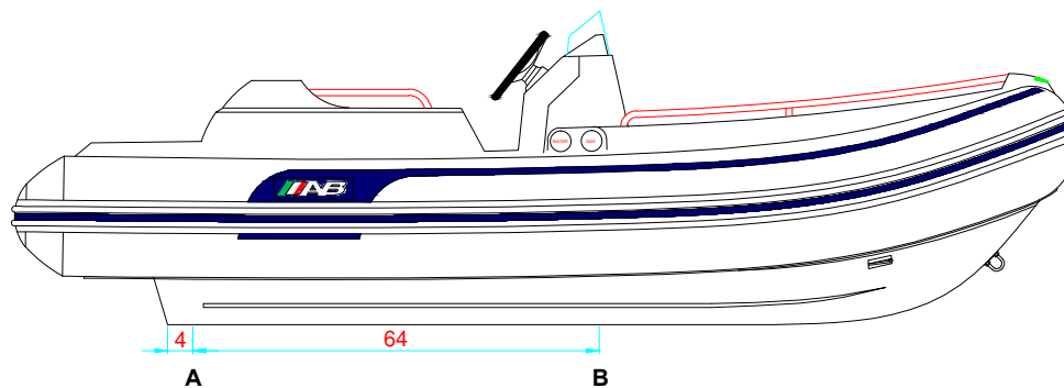
LONGITUDINAL PROFILE VISTA LATERAL
