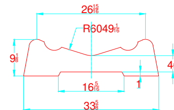
TRANSVERSAL SECTION "B" SECCION TRANSVERSAL "B"
