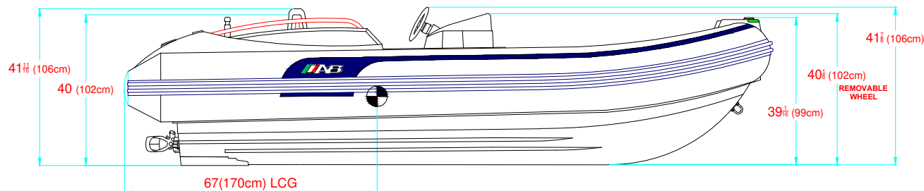
LONGITUDINAL PROFILE VISTA LATERAL
