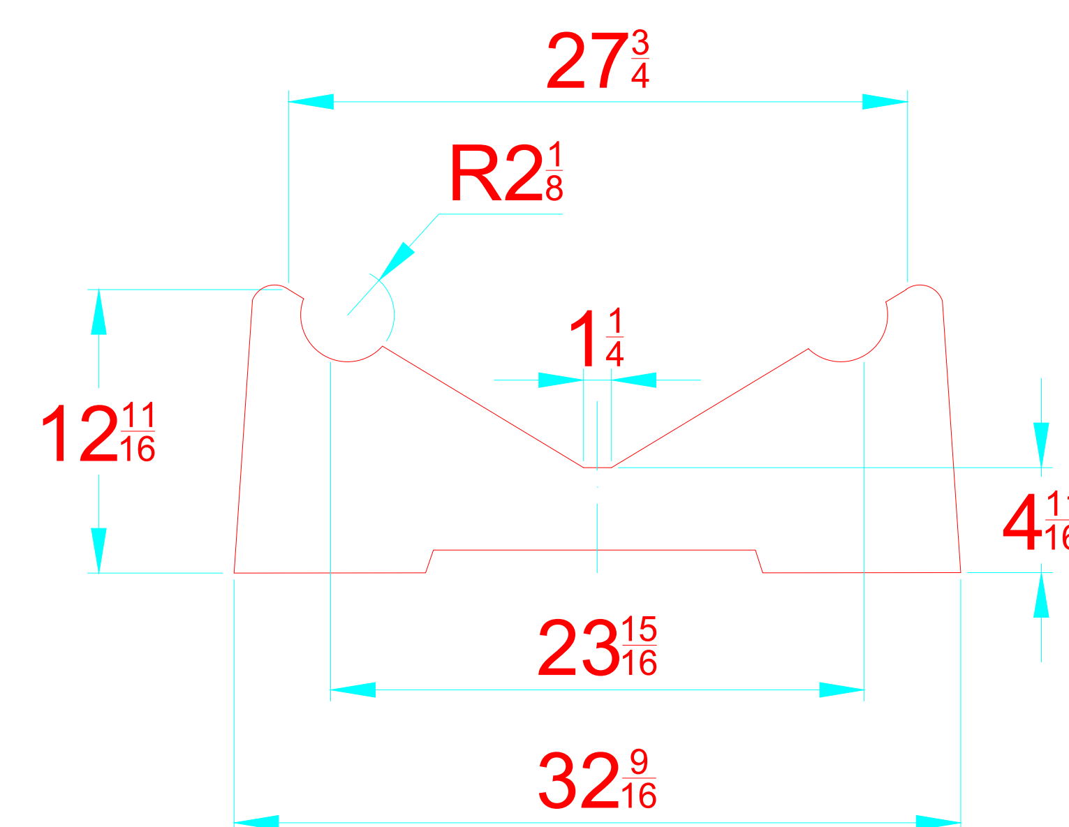
TRANSVERSAL SECTION "B" SECCION TRANSVERSAL "B"
