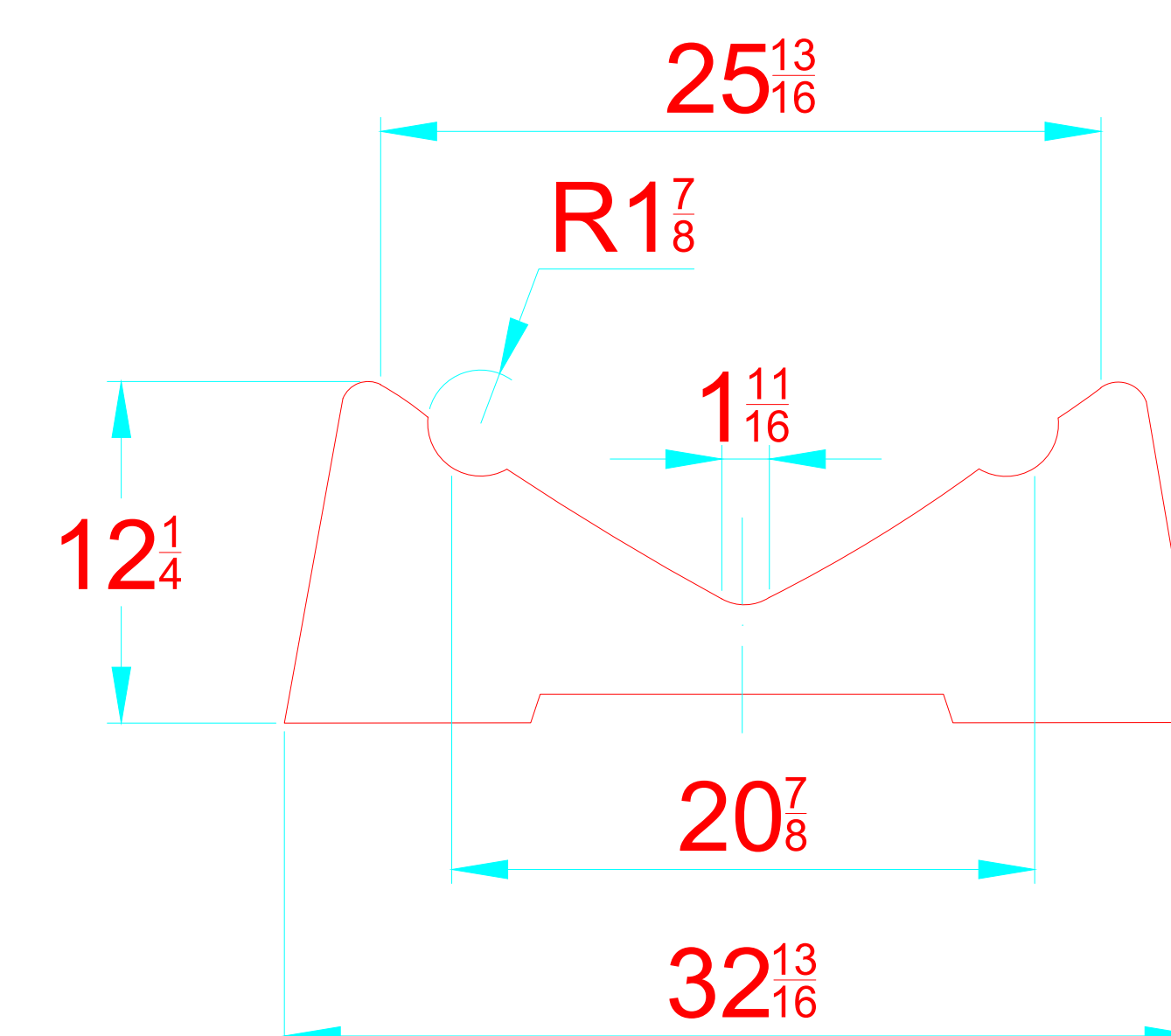
TRANSVERSAL SECTION "B" SECCION TRANSVERSAL "B"
