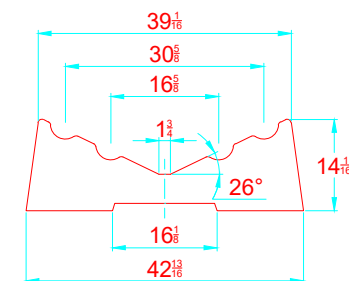
TRANSVERSAL SECTION "B" SECCION TRANSVERSAL "B"
