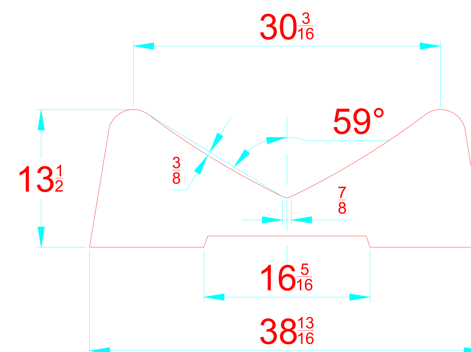
TRANSVERSAL SECTION "B" SECCION TRANSVERSAL "B"
