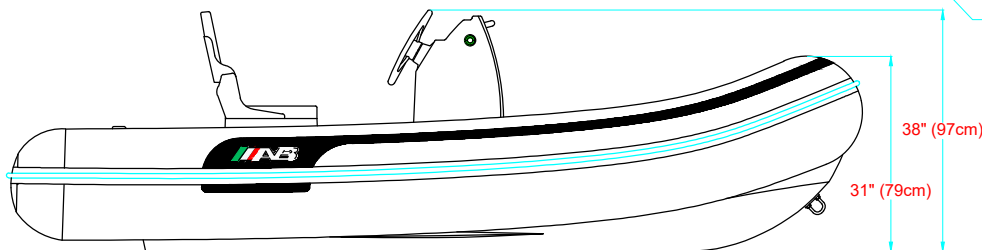
VISTA LATERAL LONGITUDINAL PROFILE
