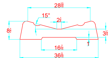
TRANSVERSAL SECTION "B" SECCION TRANSVERSAL "B"
