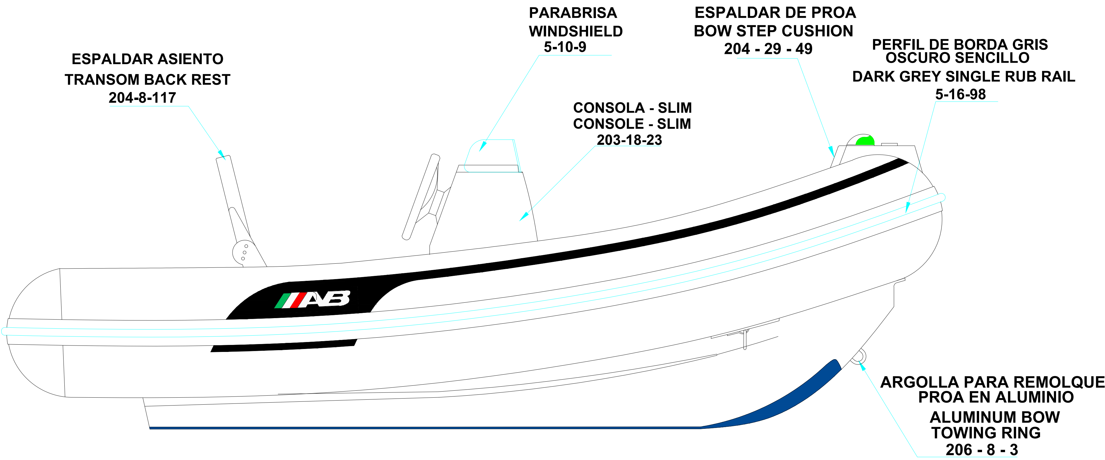
LONGITUDINAL PROFILE VISTA LATERAL
