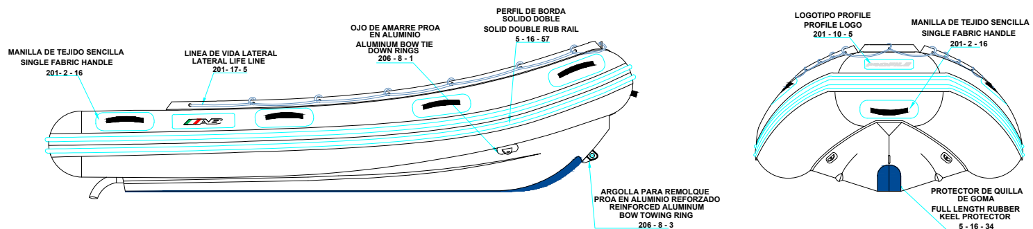
LONGITUDINAL PROFILE VISTA LATERAL
