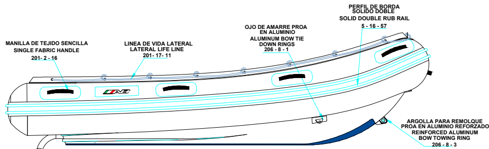
LONGITUDINAL PROFILE VISTA LATERAL
