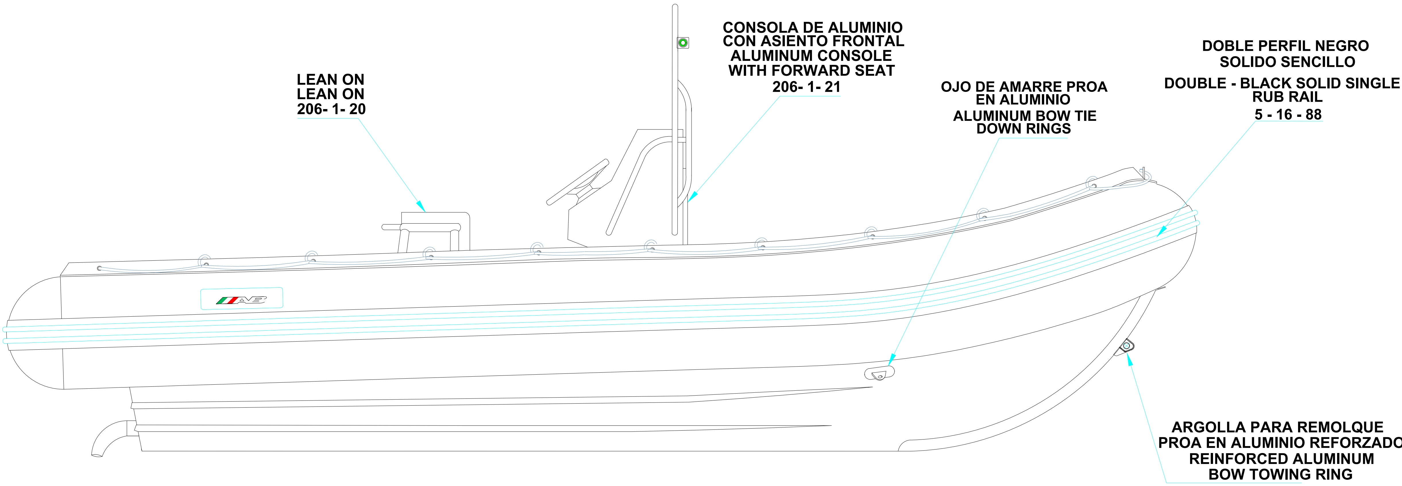
LONGITUDINAL PROFILE VISTA LATERAL
