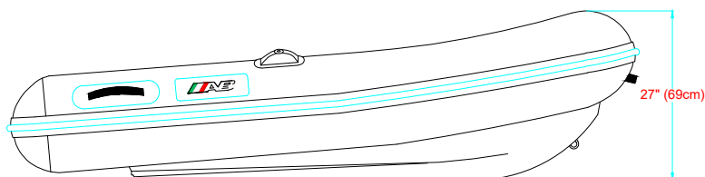
LONGITUDINAL PROFILE VISTA LATERAL
