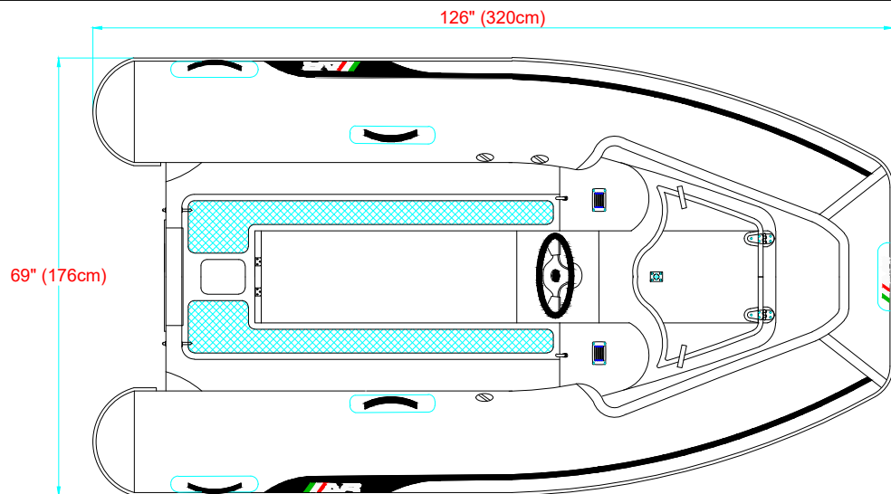
PLANT VIEW VISTA EN PLANTA
