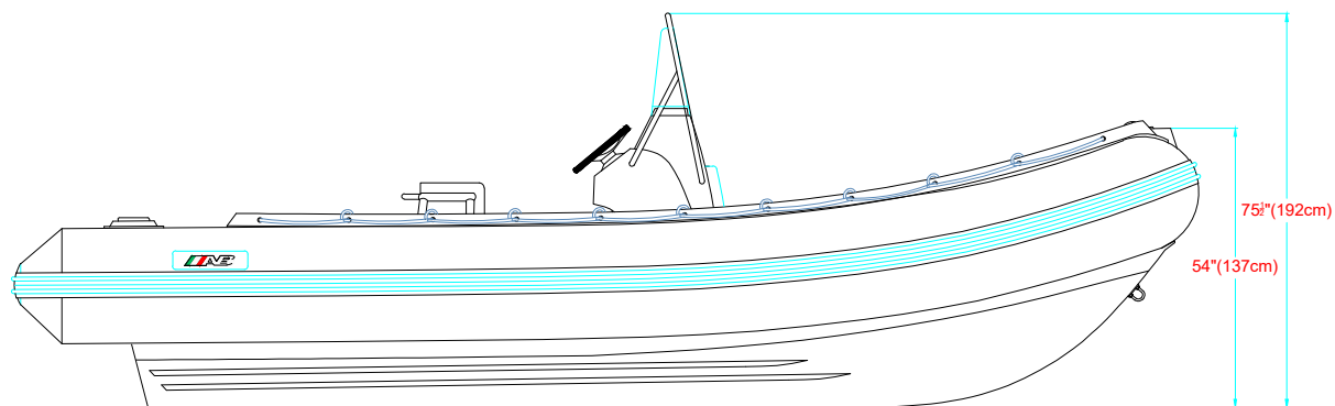
LONGITUDINAL PROFILE VISTA LATERAL
