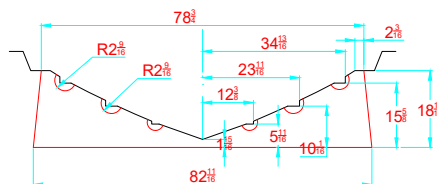
TRANSVERSAL SECTION "B" SECCION TRANSVERSAL "B"
