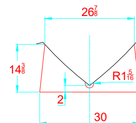
TRANSVERSAL SECTION "B" SECCION TRANSVERSAL "B"
