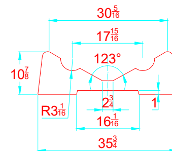
TRANSVERSAL SECTION "B" SECCION TRANSVERSAL "B"
