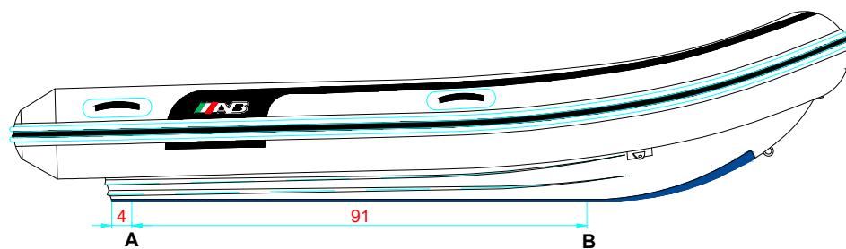
LONGITUDINAL PROFILE PERFIL LONGITUDINAL
