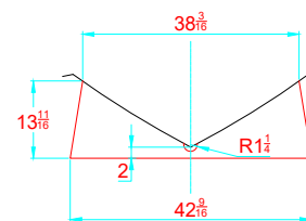
TRANSVERSAL SECTION "B" SECCION TRANSVERSAL "B"
