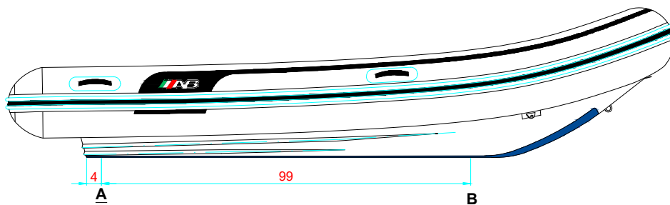
LONGITUDINAL PROFILE PERFIL LONGITUDINAL
