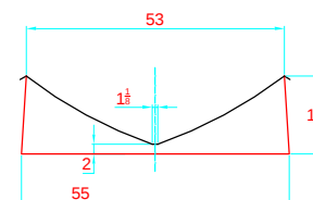
TRANSVERSAL SECTION "B" SECCION TRANSVERSAL "B"
