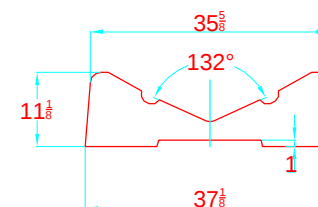
TRANSVERSAL SECTION "B" SECCION TRANSVERSAL "B"
