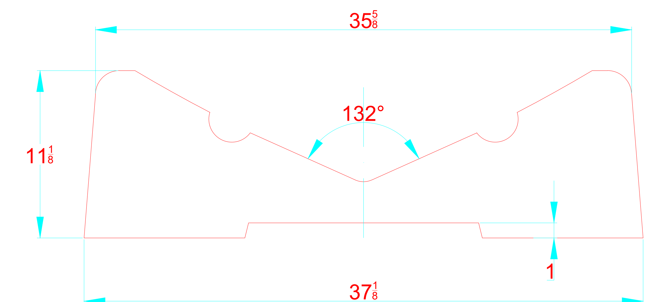
TRANSVERSAL SECTION "B" SECCION TRANSVERSAL "B"
