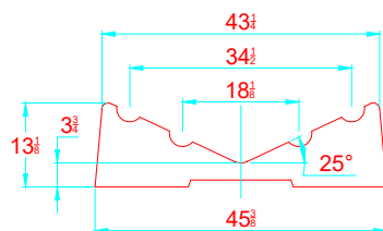
TRANSVERSAL SECTION "B" SECCION TRANSVERSAL "B"
