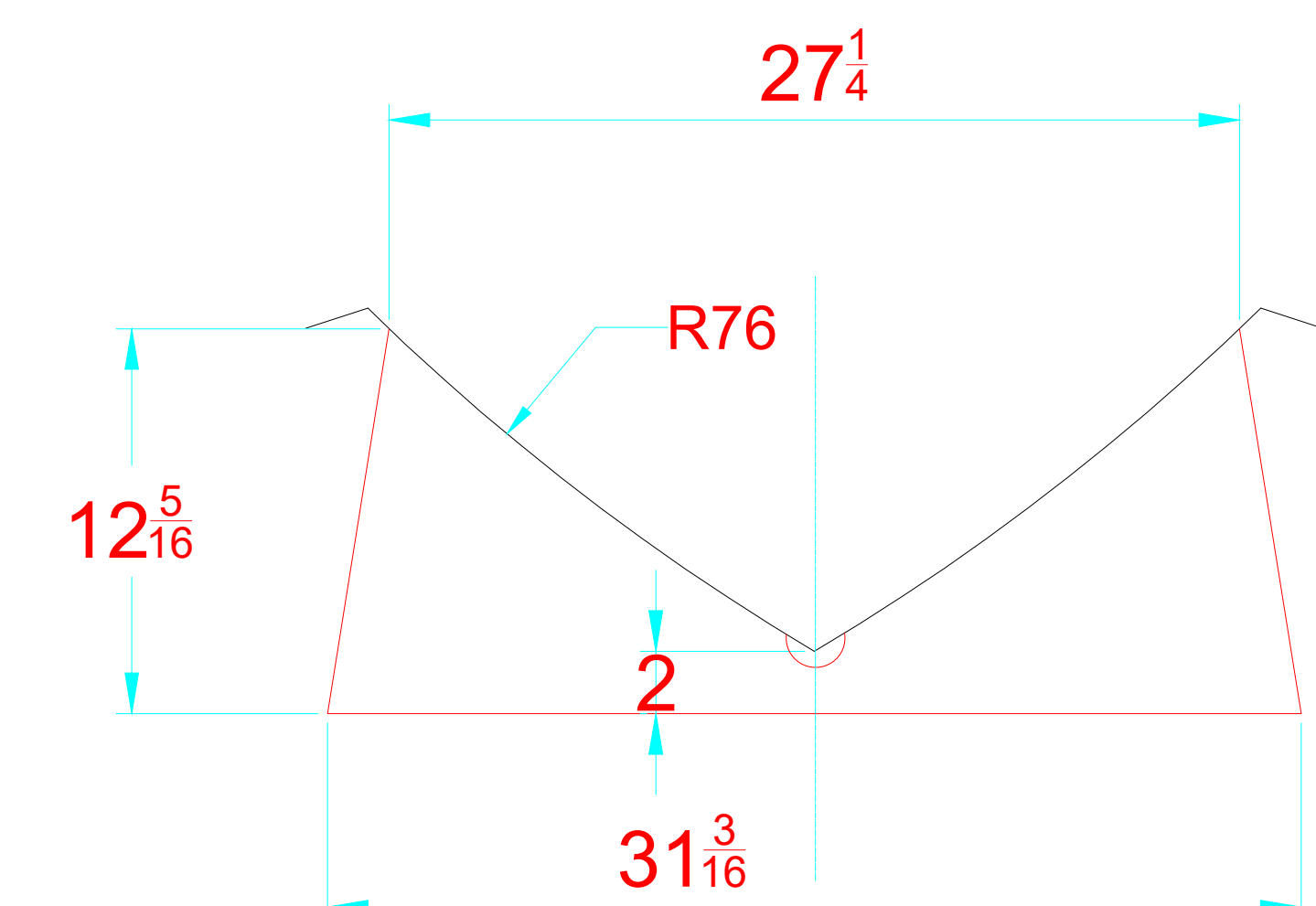
TRANSVERSAL SECTION "B" SECCION TRANSVERSAL "B"
