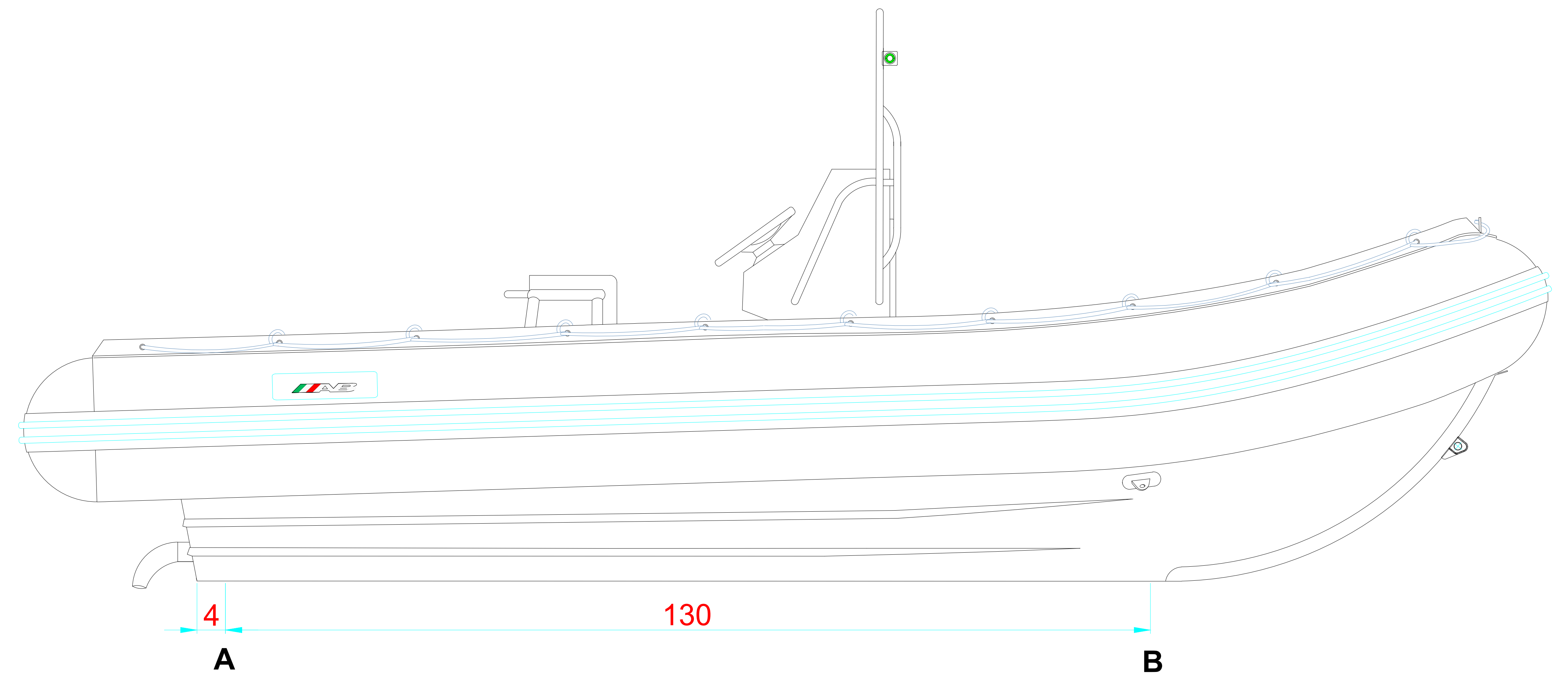
LONGITUDINAL PROFILE PERFIL LONGITUDINAL
