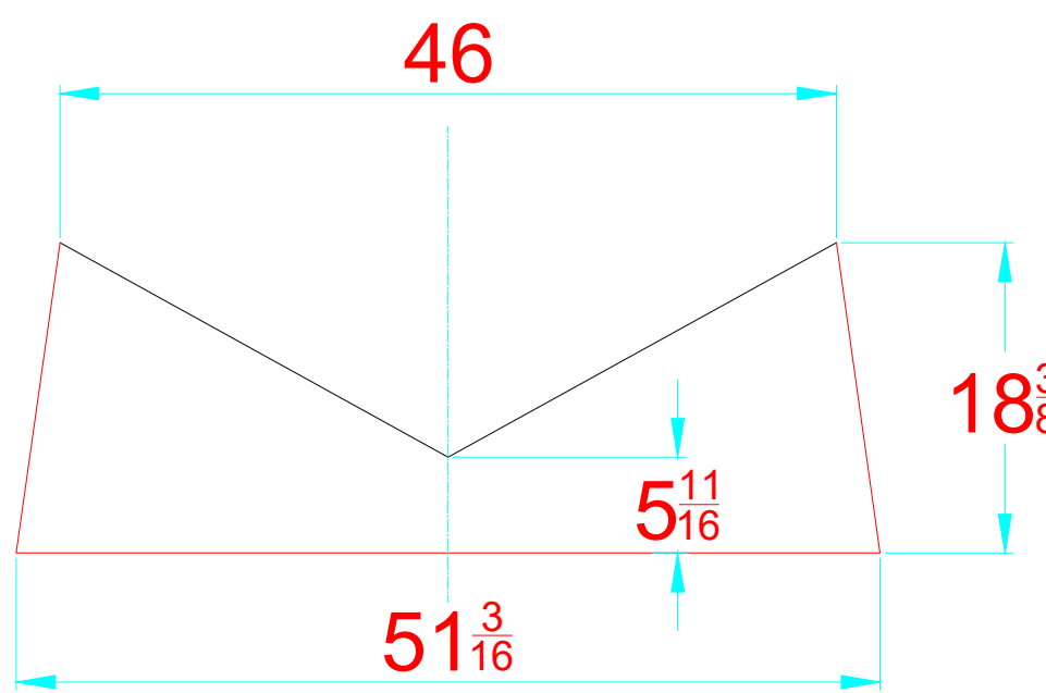
TRANSVERSAL SECTION "B" SECCION TRANSVERSAL "B"
