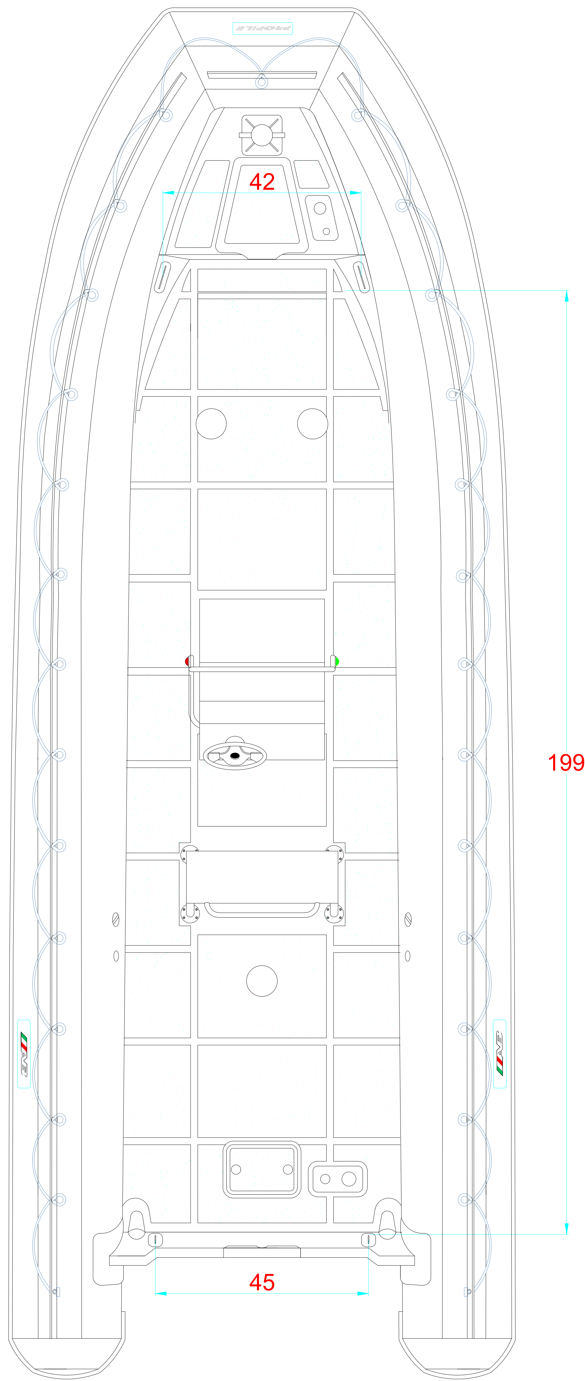
-LOCATION AND DISTANCE OF DAVIT LIFTING POINTS UBICACION Y DISTANCIA DE LOS GANCHOS DE IZADO
