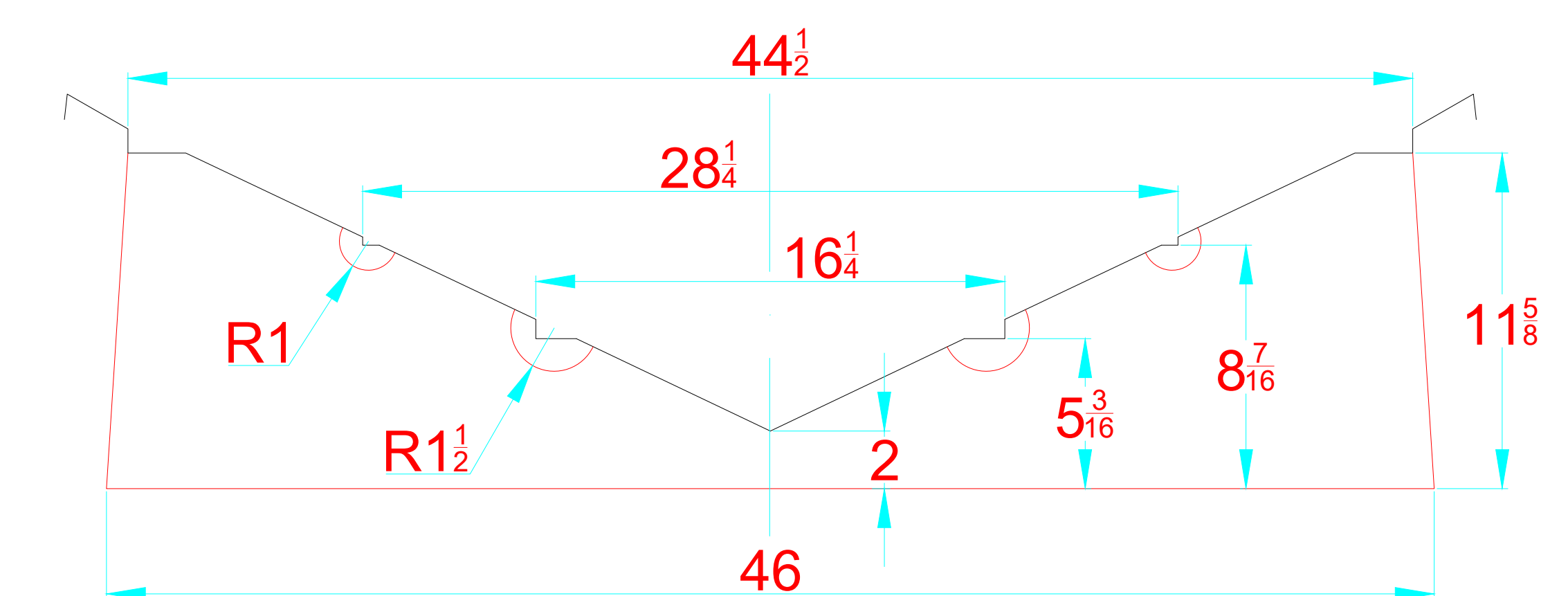
TRANSVERSAL SECTION "B" SECCION TRANSVERSAL "B"
