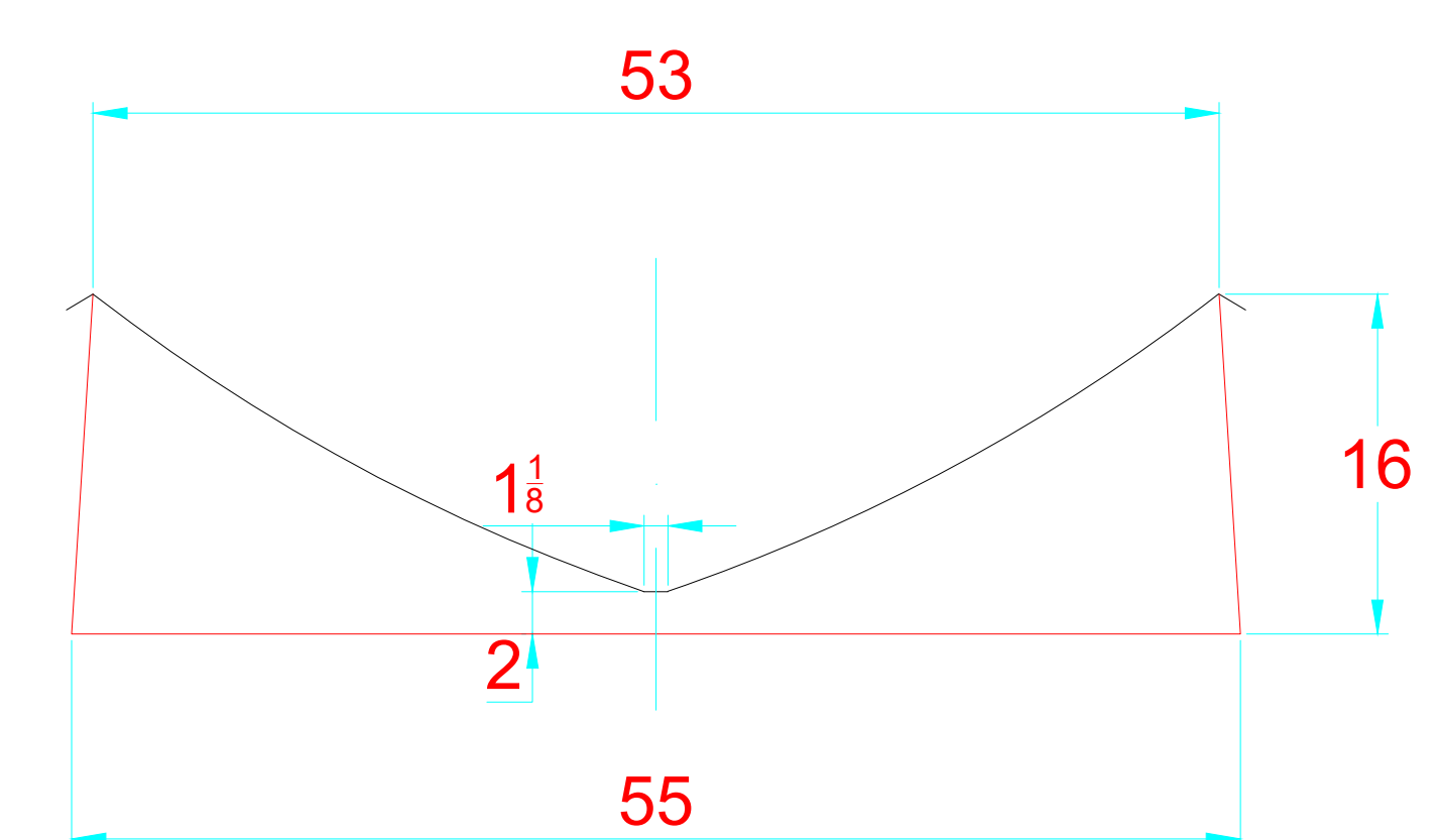
TRANSVERSAL SECTION "B" SECCION TRANSVERSAL "B"
