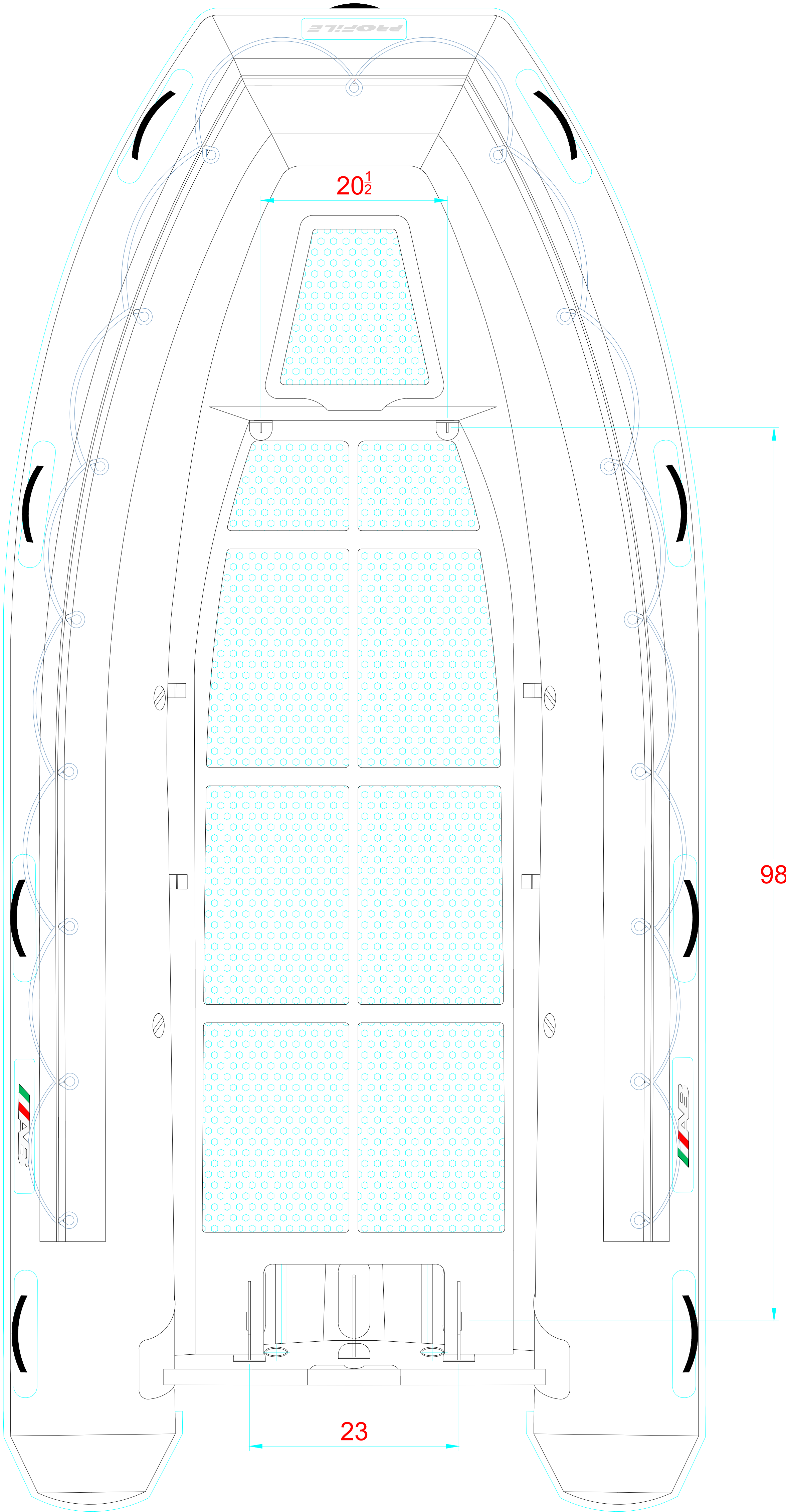
-LOCATION AND DISTANCE OF DAVIT LIFTING POINTS UBICACION Y DISTANCIA DE LOS GANCHOS DE IZADO
